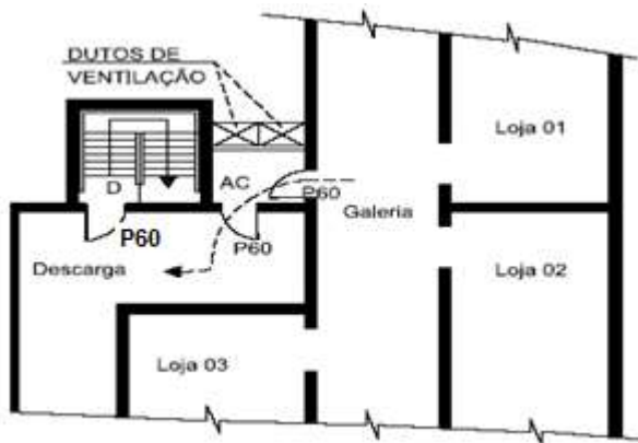
Figura 25 – Acesso de galeria comercial à descarga
