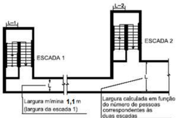
Figura 24 – Dimensionamento de corredores de descargada
