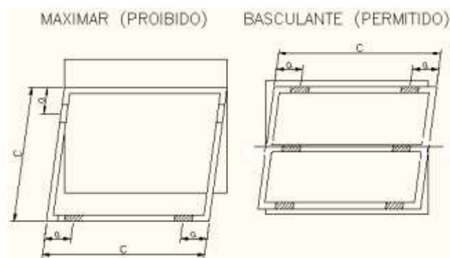
Figura 10 – Janela da escada enclausurada protegida
