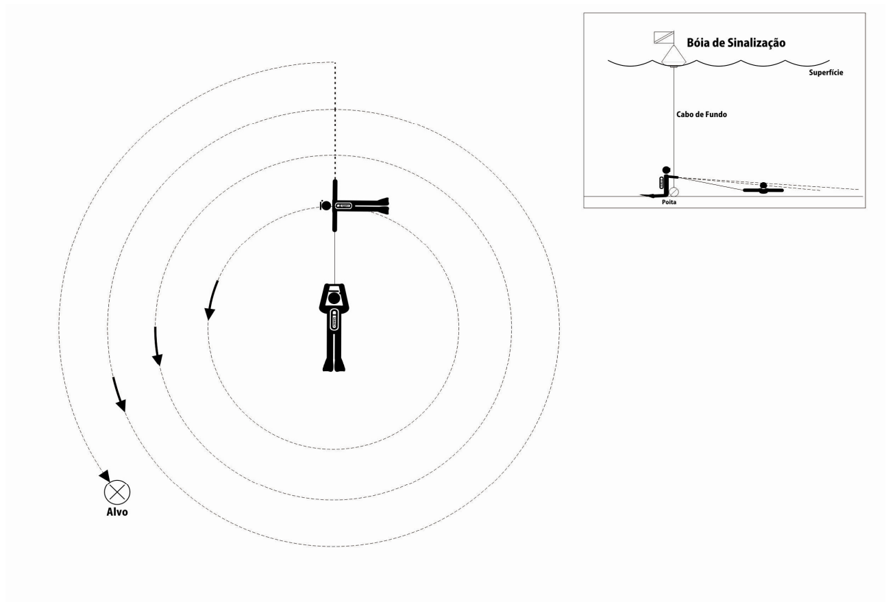
Figura 07 – Busca circular.
