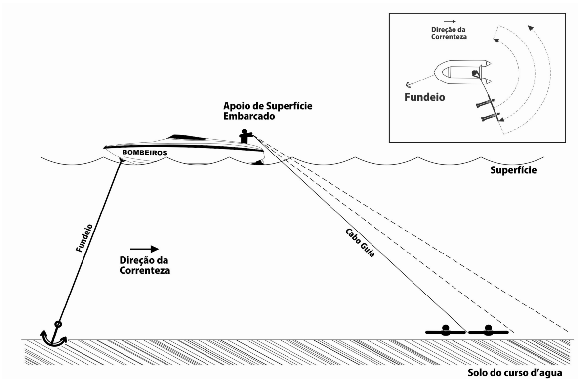
Figura 04 – Busca semicircular com apoio de superfície embarcado.
